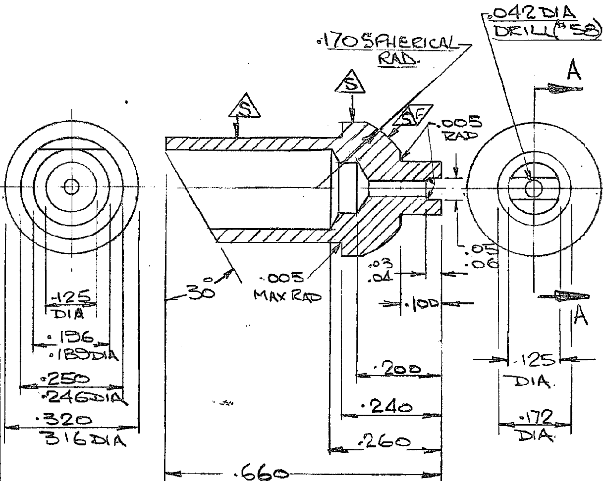
SECTION A-A
